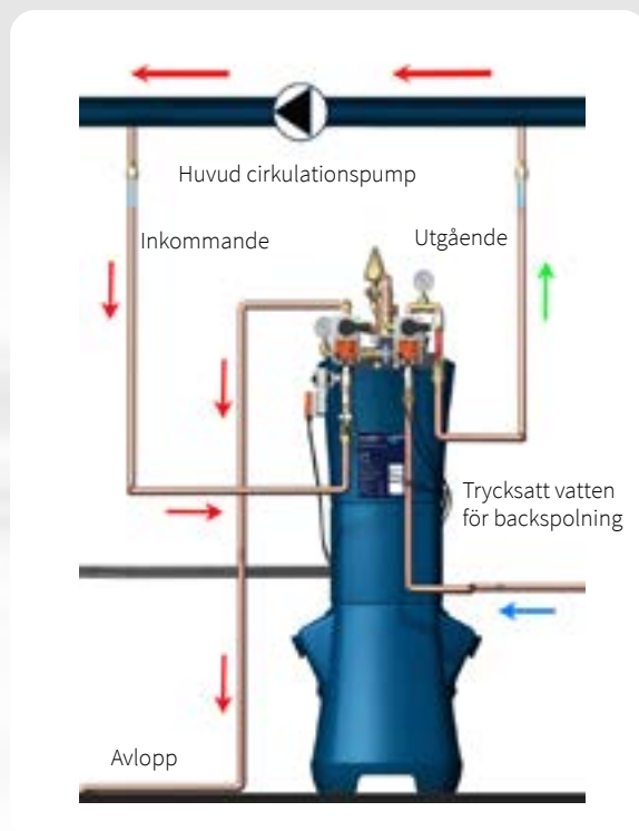
Installationsexempel
